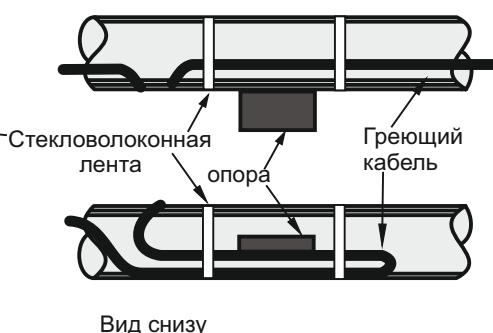
Рис.2 Опора трубы
